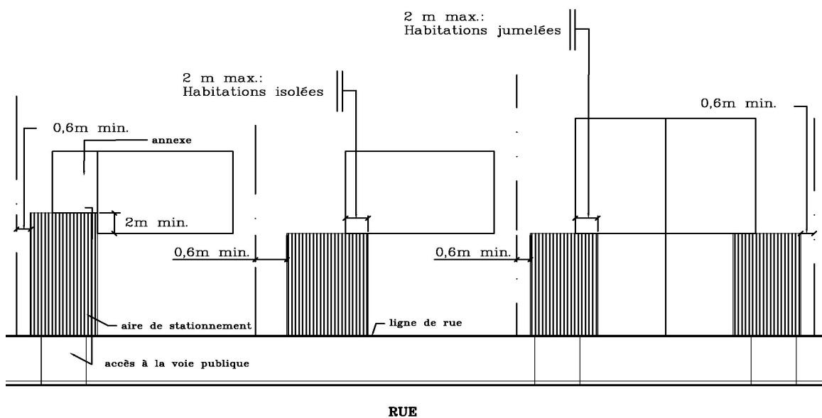
Figures 6 - Normes d'implantation et de dimensions d'une aire de stationnement pour une habitation isolée ou jumelée de 3 logements et plus
